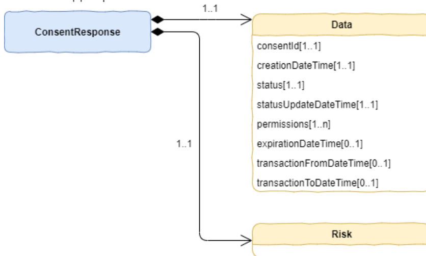
Рисунок 6 - Диаграмма объекта ConsentResponse
