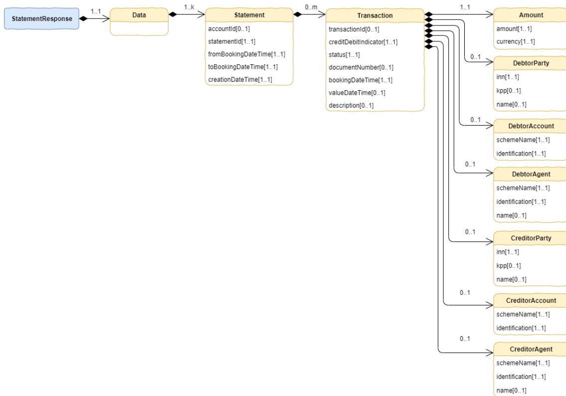
Рисунок 13 - Диаграмма объекта StatementResponse
