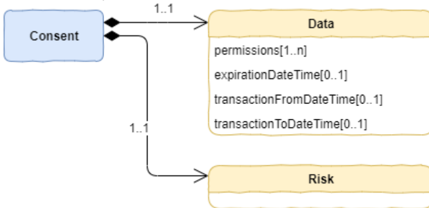
Рисунок 5 - Диаграмма объекта Consent
