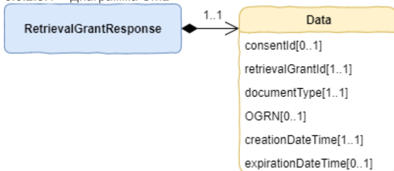
Рисунок 7 - Диаграмма объекта RetrievalGrantResponse
