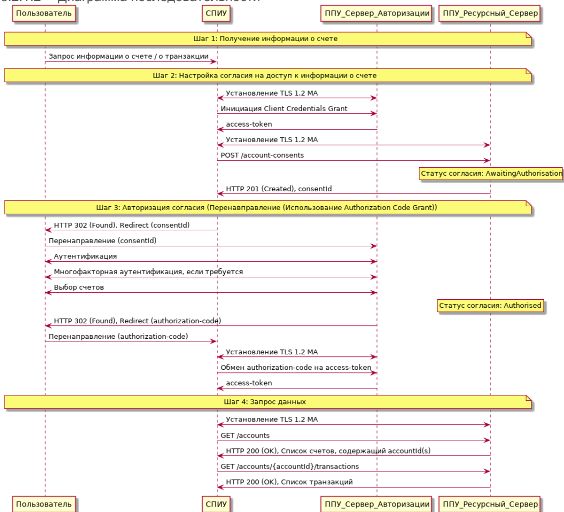
Рисунок 2 - Диаграмма последовательности для получения информации о счете
