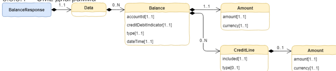
Рисунок 9 - Диаграмма объекта BalanceResponse
