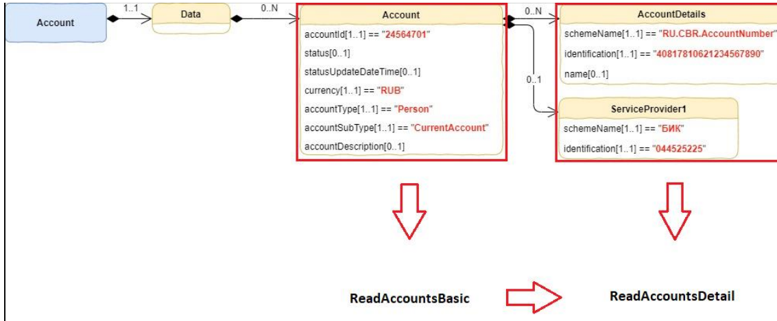
Рисунок 3 - Пример применения базового и детального разрешений на доступ к кластерам данных
