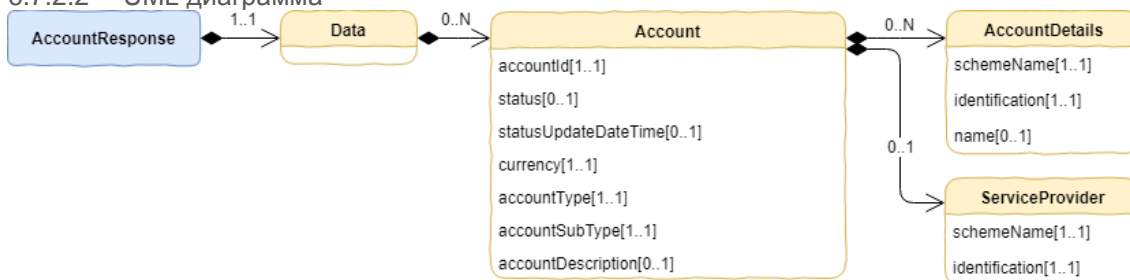
Рисунок 8 - Диаграмма объекта AccountResponse
