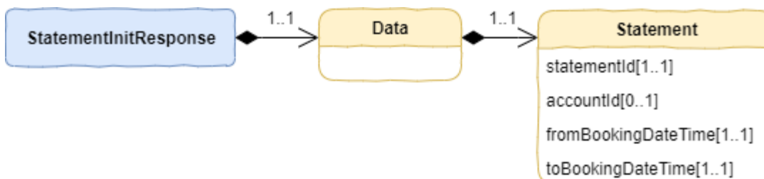
Рисунок 12 - Диаграмма объекта StatementInitResponse
