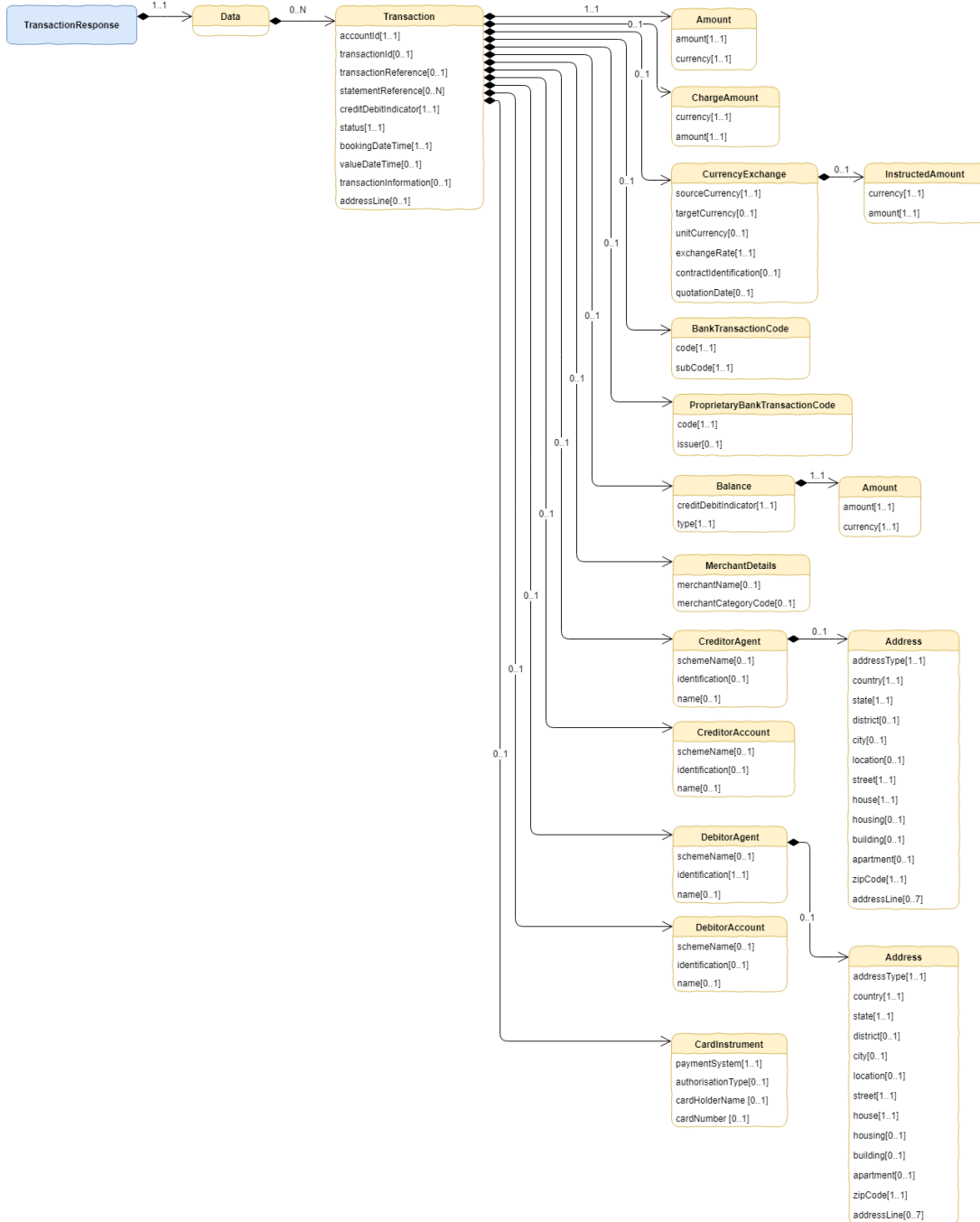
Рисунок 10 - Диаграмма объекта TransactionResponse
