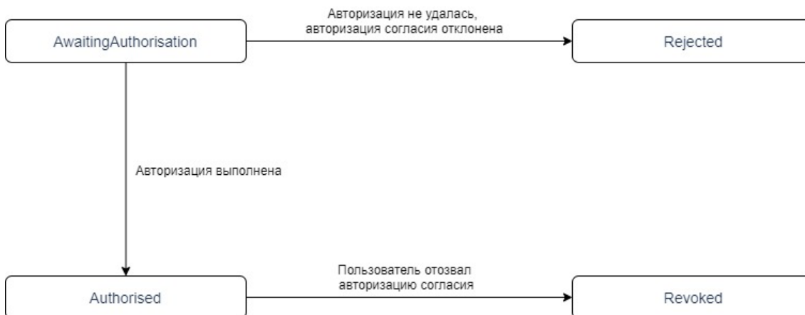
Рисунок 4 - Диаграмма состояний ресурса согласия на доступ к счету
